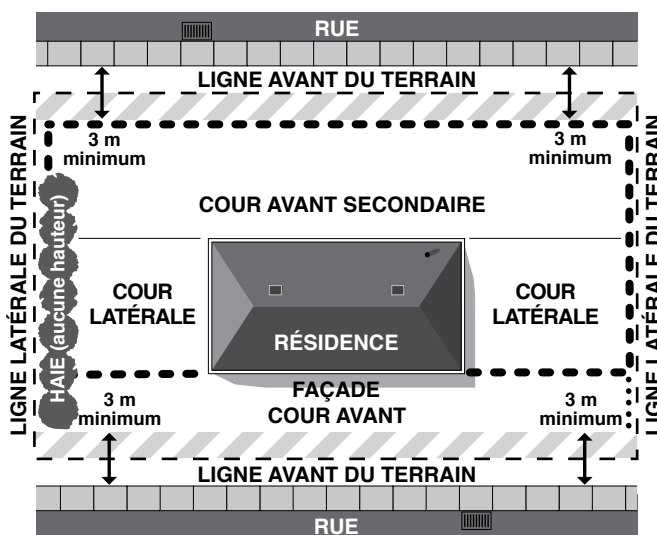
CROQUIS 3 – INSTALLATION SUR UN TERRAIN TRANSVERSAL
